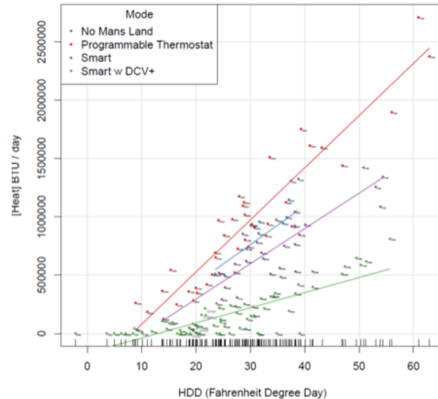
GTI North Zone - actual energy consumed
